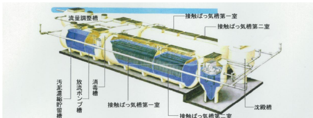
図1 工場製作型極小規模処理施設（接触酸化型）イメージ図
