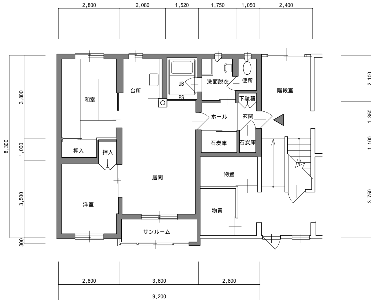
川添2LDK (H5) tomato東階段室
