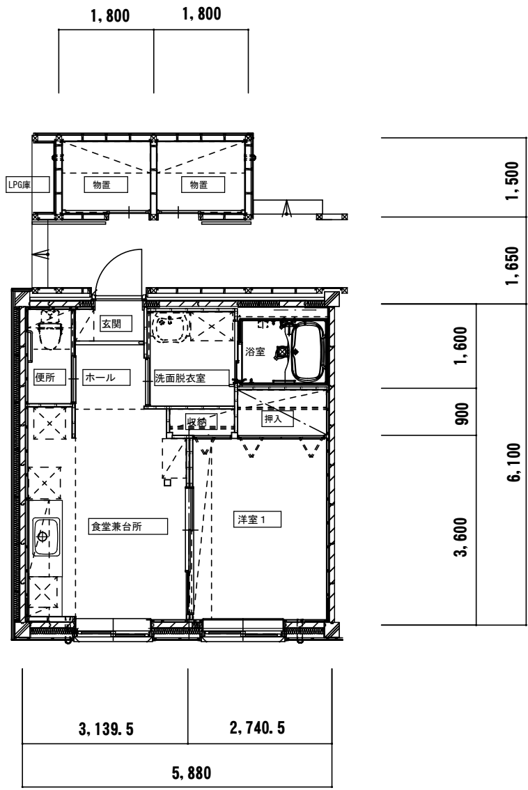
西団地A棟 1DK
